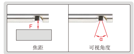
侧视(装上90°反光镜后)
